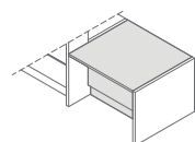
LAU21L 1000 / 917 / 740 29.5 kg
