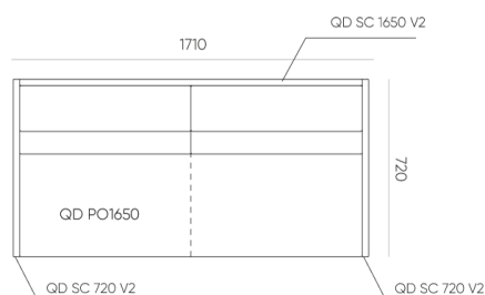
QD PO 1650 + QD SC 1650 V2 + 2X QD SC 720 V2
