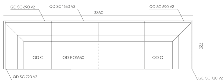
QD PO 1650 +2X QD C + 2X QD SC 720 V2+ 2X QD SC 690 V2 + QD SC 1650 V2
