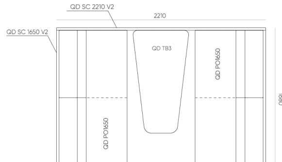
QD BOX (2X QD PO 1650 + 2X QD SC 1650 V2 + QD SC 2210 V2 + QD TB3)
