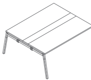
SW46L 1600 / 1410 / 740 65.4 kg
