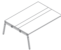
SW48L 1800 / 1410 / 740 73.3 kg
