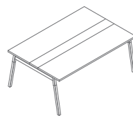
SW28 1800 / 1210 / 740 72.6 kg
