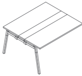
SW24L 1400 / 1210 / 740 53.95 kg
