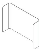
AP01 1220 / 290 / 880 10.8 kg
